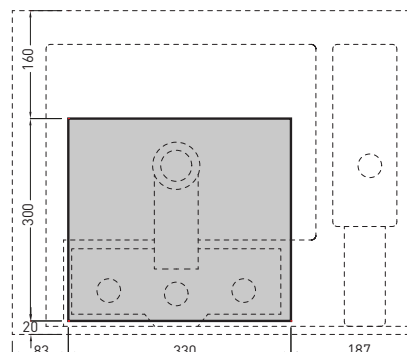
FORO SU PIANO OPZIONE 1 ON TOP HOLE OPTION 1
